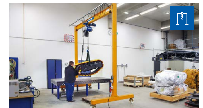
Portiques légers LPK
