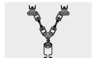
Suspension en V
